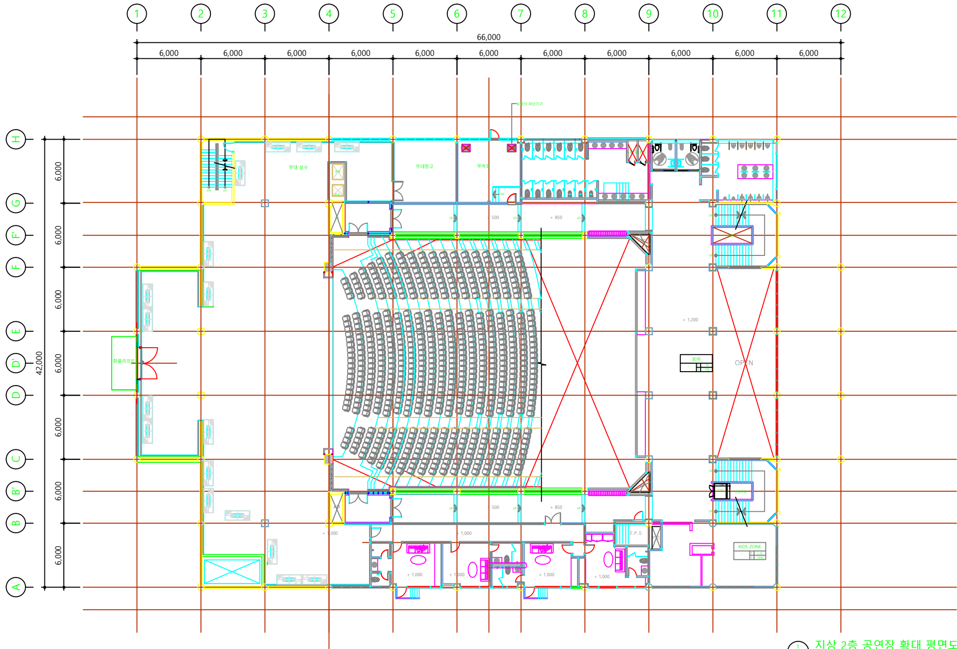
1 지상 2층 공연장 확대 평면도 AR-010 SCALE : 1/250
